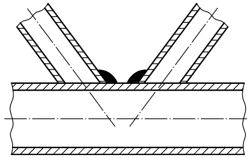
Getrennte Bauteile Nicht überlappende Schweißnähte EMPFOHLENE AUSFÜHRUNG
