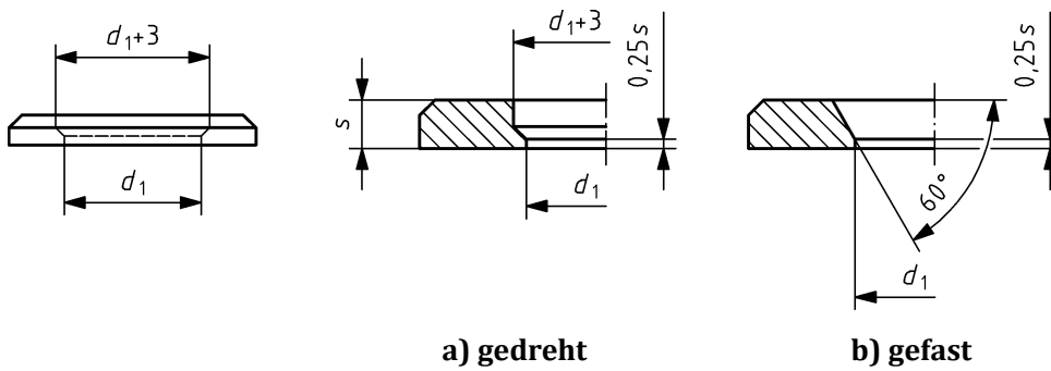
Bild J.3 — Vorbereitung der Scheibe zum Einsatz unter dem Schraubenkopf
