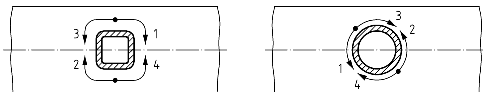
Bild E.1 — Nahtanfangs- und Nahtendstellen und Schweißfolge
