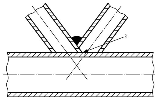
Getrennte Bauteile Nicht überlappende Schweißnähte EMPFOHLENE AUSFÜHRUNG
