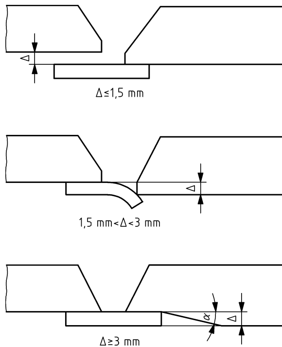
Bild E.8 — Schweißbadsicherungsdetails für Bauteile unterschiedlicher Dicke
