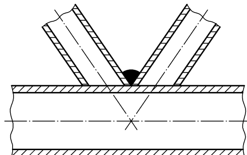
Getrennte Bauteile aber überlappende Schweißnähte ZU VERMEIDENDE AUSFÜHRUNG
