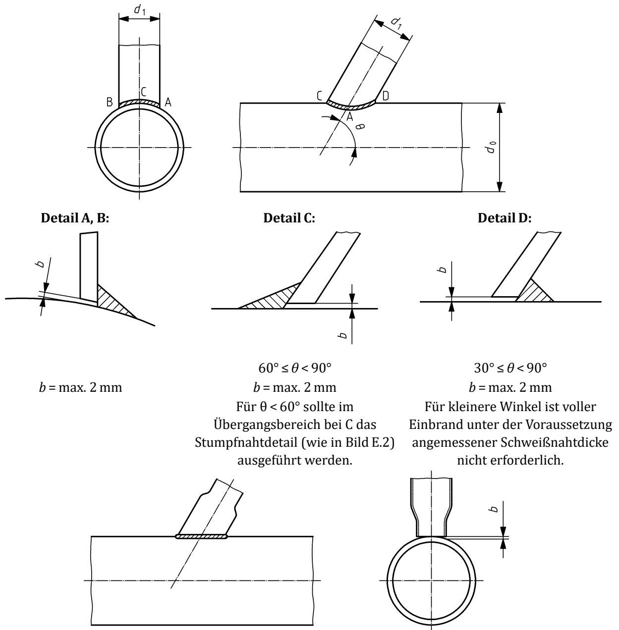
Bild E.3 — Nahtvorbereitung und Passgenauigkeit von Kehlnähten bei Gurt-Streben-Anschlüssen von kreisförmigen Hohlprofilen
