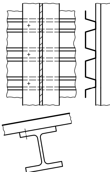
b) I-Profil bei einseitiger Anordnung, nur bei geneigtem Dach zulässig
