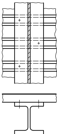
a) I-Profil bei alternierender Anordnung
