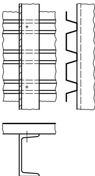
a) I-Profil bei alternierender Anordnung
