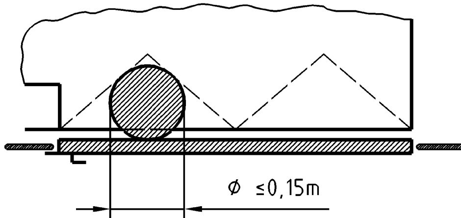
Bild 6 — Abstand zwischen Schacht-Drehtür und Fahrkorb-Falztür
