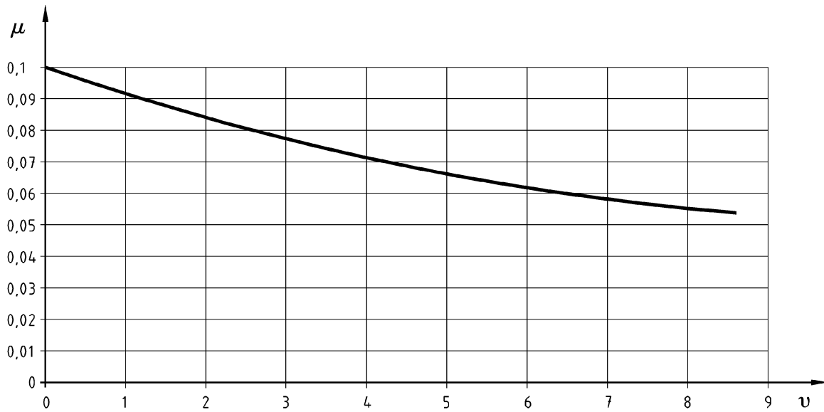
Bild K.3 — Mindest erforderliche Reibungszahl
