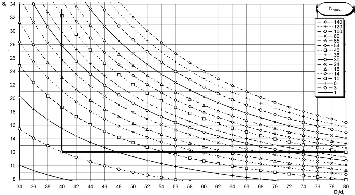
Bild L.1 — Bestimmung des minimalen Sicherheitsbeiwertes
