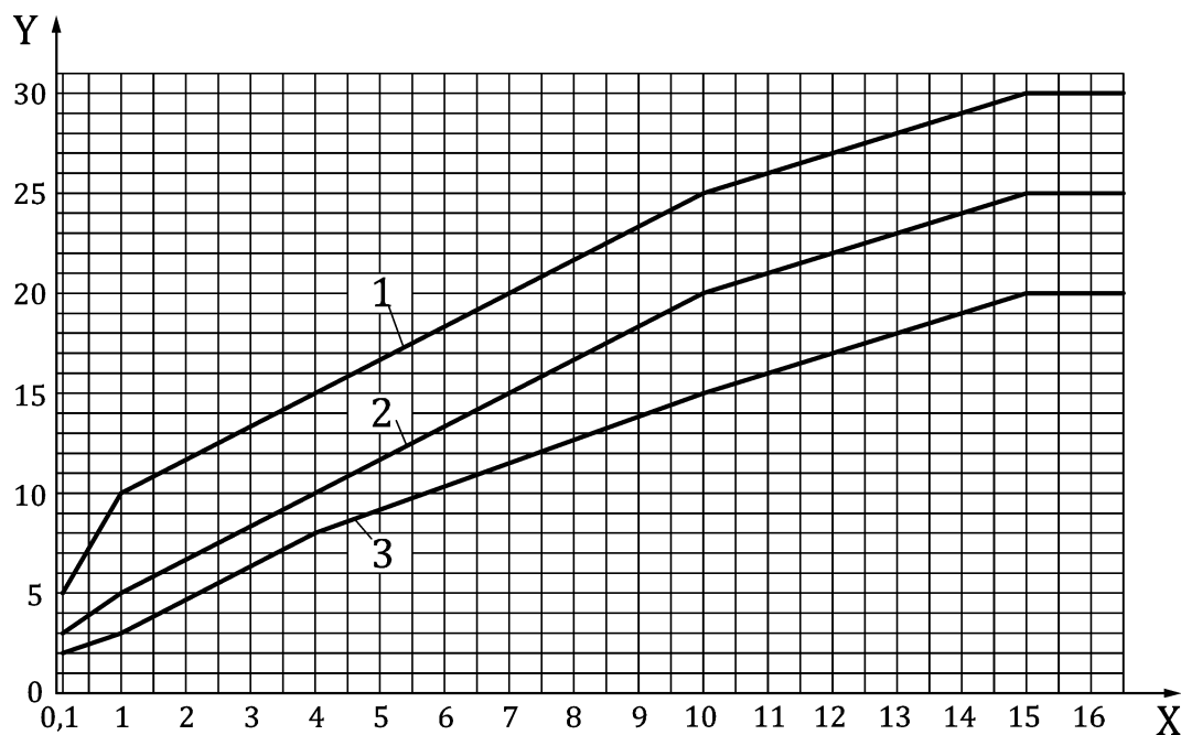
Bild 6 — Grenzwerte für Ebenheitsabweichungen von Oberseiten von Decken, Estrichen und Fußböden (Angabe der Zeilen nach Tabelle 3)
