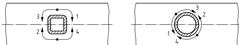
Bild E.1 — Nahtanfangs- und Nahtendstellen und Schweißfolge
