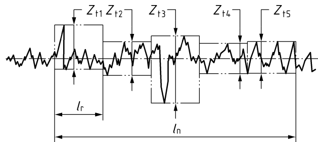
Bild D.3 — Bestimmung der gemittelten Rautiefe R_{Z5}
