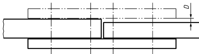
Bild 3 — Dickenunterschied von Bauteilen in der gleichen Lage
