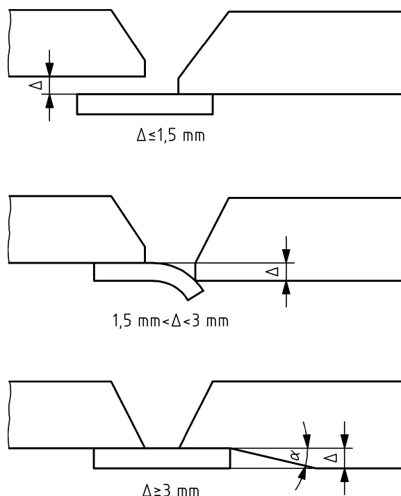
Bild E.8 — Schweißbadsicherungsdetails für Bauteile unterschiedlicher Dicke
