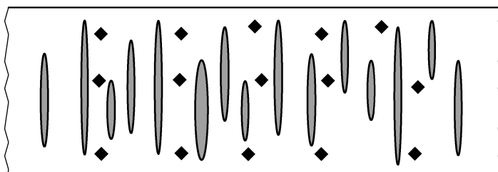
Bild D.4 — Messstellen auf der geschliffenen Brennschnittoberfläche
