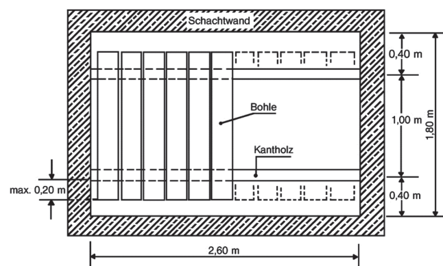
Abb. C1: Stützweite der Kanthölzer in Längsrichtung
