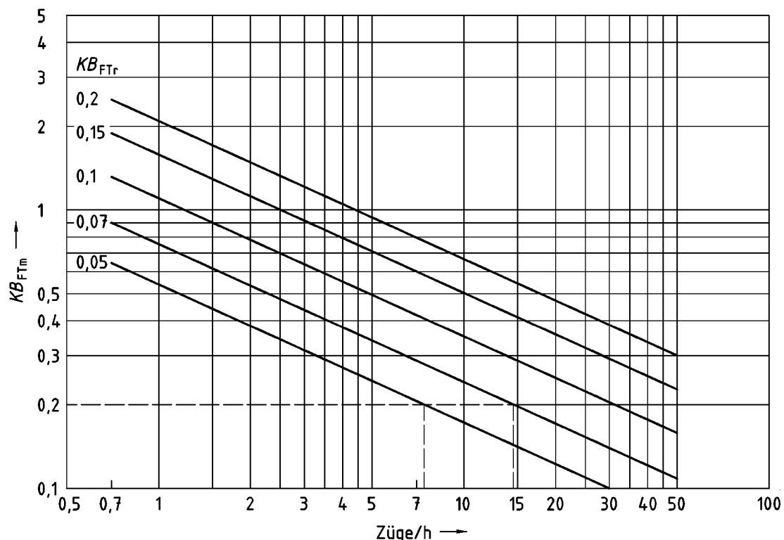
Bild D.1: Zusammenhang zwischen der Beurteilungs-Schwingstärke KB_{FTT} , dem Taktmaximal-Effektivwert KB_{FTM} und der Zughäufigkeit (Annahmen: Nur eine Zugklasse, und jeder Zug belegt nur einen Takt.)
