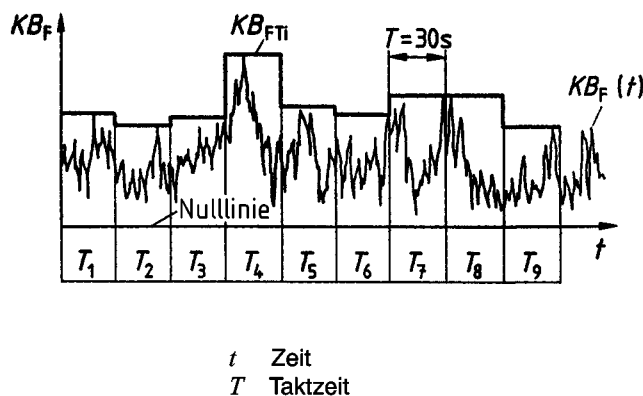
Bild 1: Ermittlung der Taktmaximalwerte KB_{FTi}
