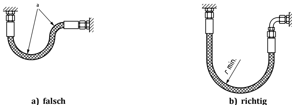
Bild 15 — Biegeradius
