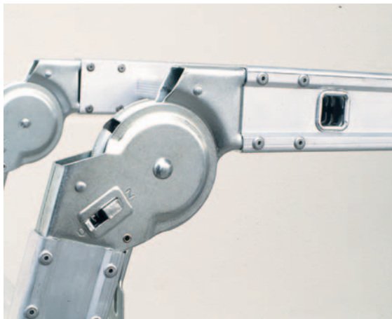
Bild 50: Sperrstellung der Gelenke
