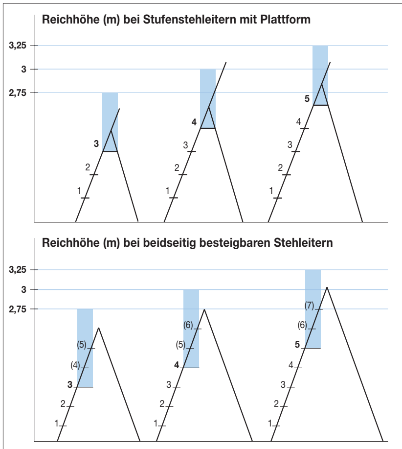
Bild 39: Reichhöhen
