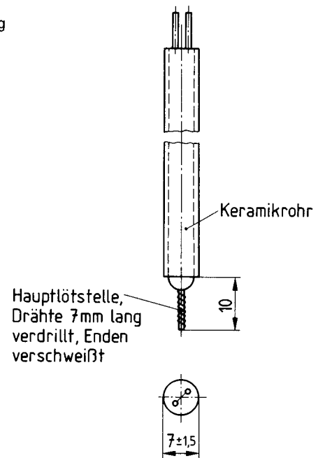
Bild 10. Thermoelemente für Rauchgastemperatur
