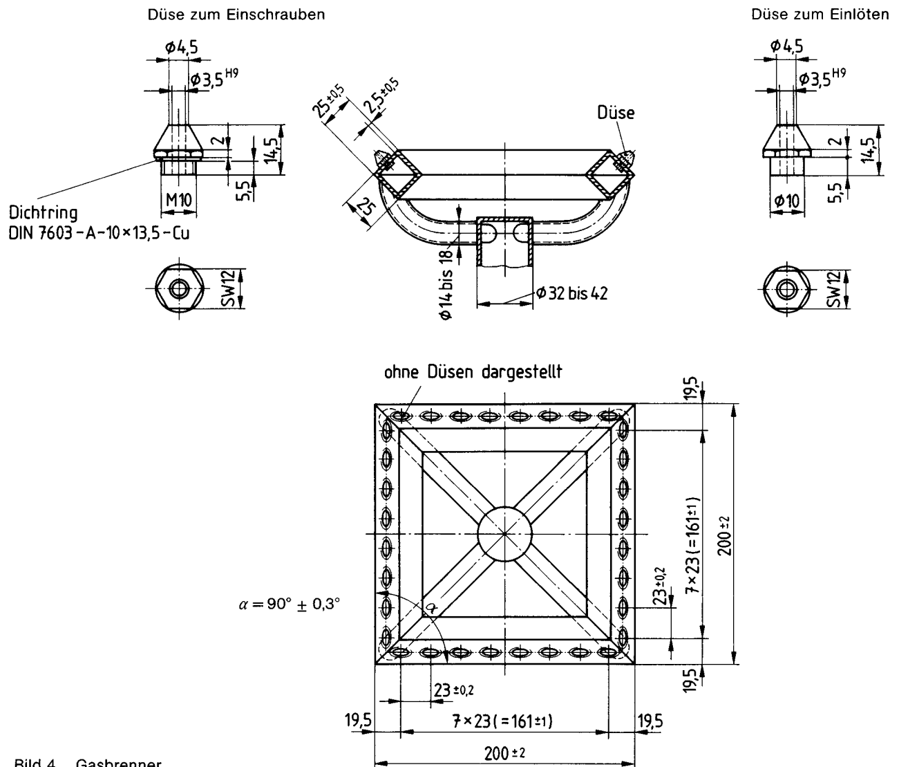
Bild 4. Gasbrenner
