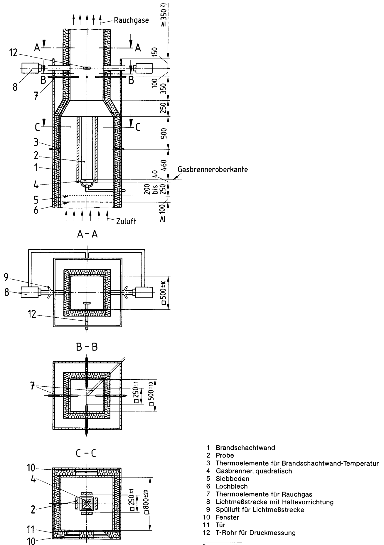
Bild 1. Brandschacht
