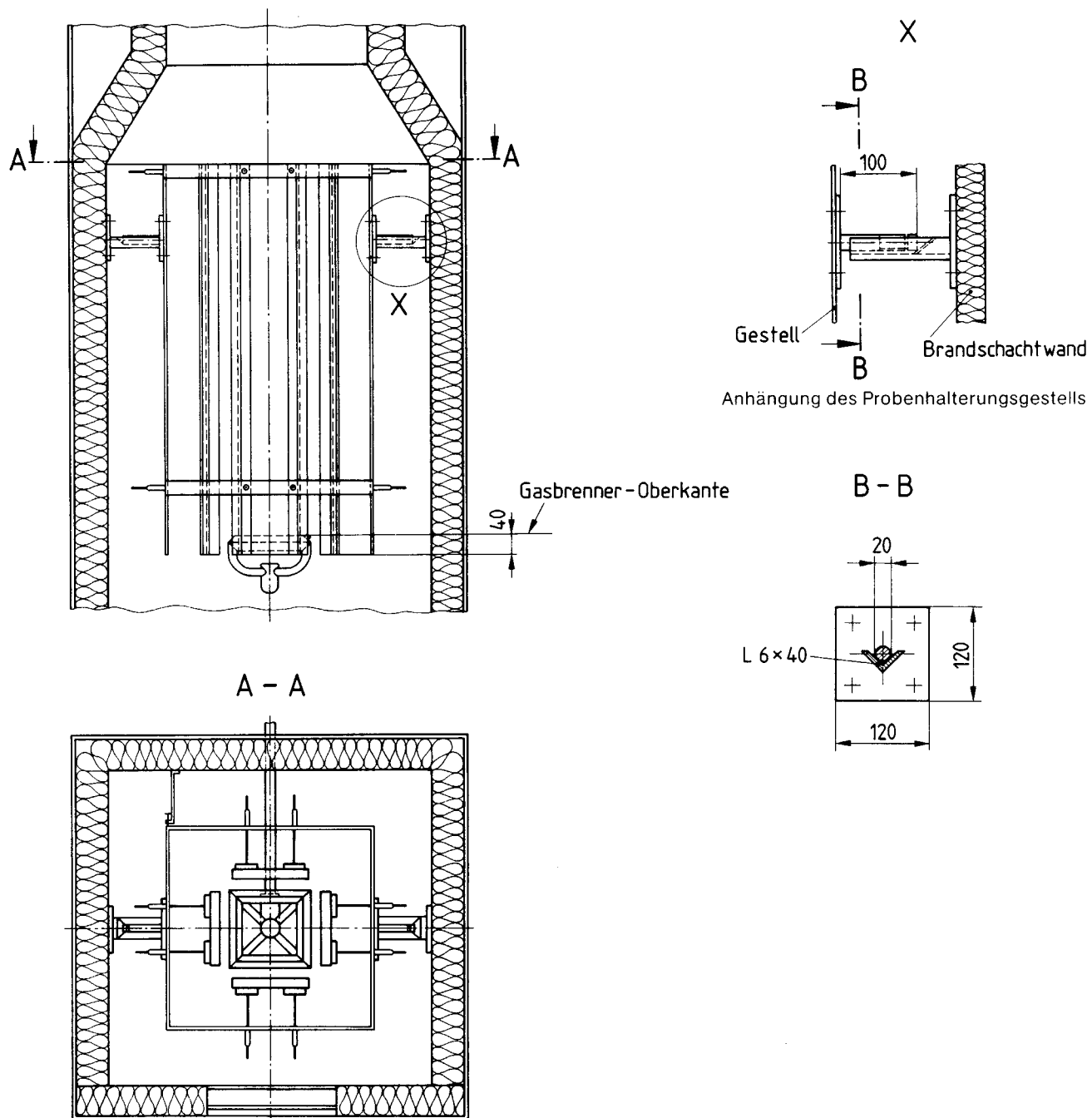
Bild 8. Beispiel für ein hängendes Gestell im Brandschacht mit Probenträgern und Proben
