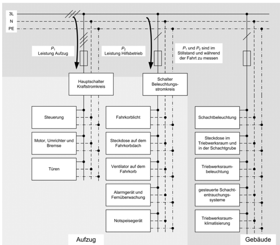
Bild 1. Ermittlung des Energiebedarfs von Aufzügen, Prinzipschaltbild
