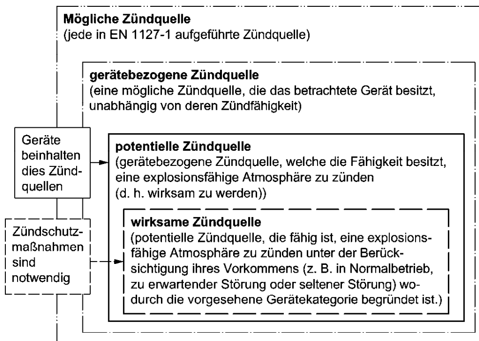
Bild 1 — Beziehung zwischen den Zündquellendefinitionen
