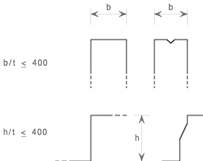
Bild 5.1 — Maximale Breite-zu-Dicke-Verhältnisse
