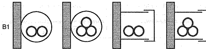
Leiter/einadrige Kabel bzw. Leitungen in Installationsrohren und in zu öffnenden Installationskanälen
