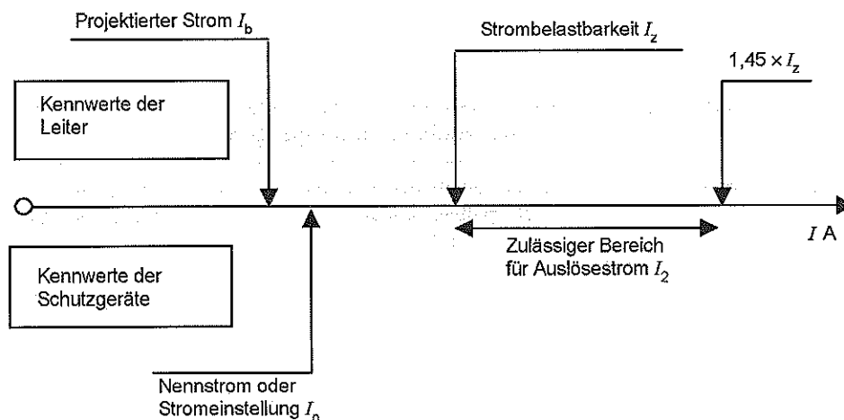
Bild D.2 – Kennwerte der Leiter und Schutzgeräte
